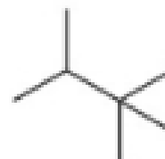
2,2,3-trimethylbutane
